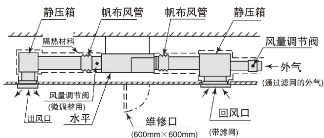
图 3.8 风管的连接
