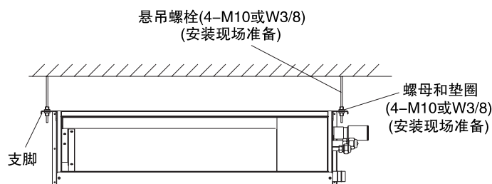
图 3.4 室内机安装
