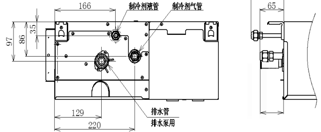
图 5.2 管连接的位置
