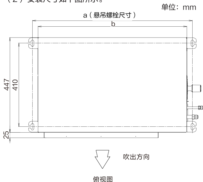
图 3.3 安装尺寸
