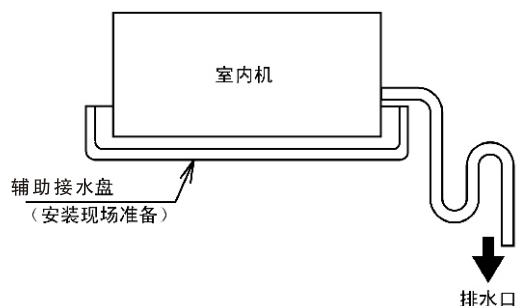
图 5.7 接水盘
