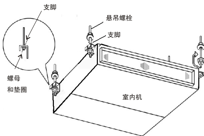
图 3.6 吊装方法
